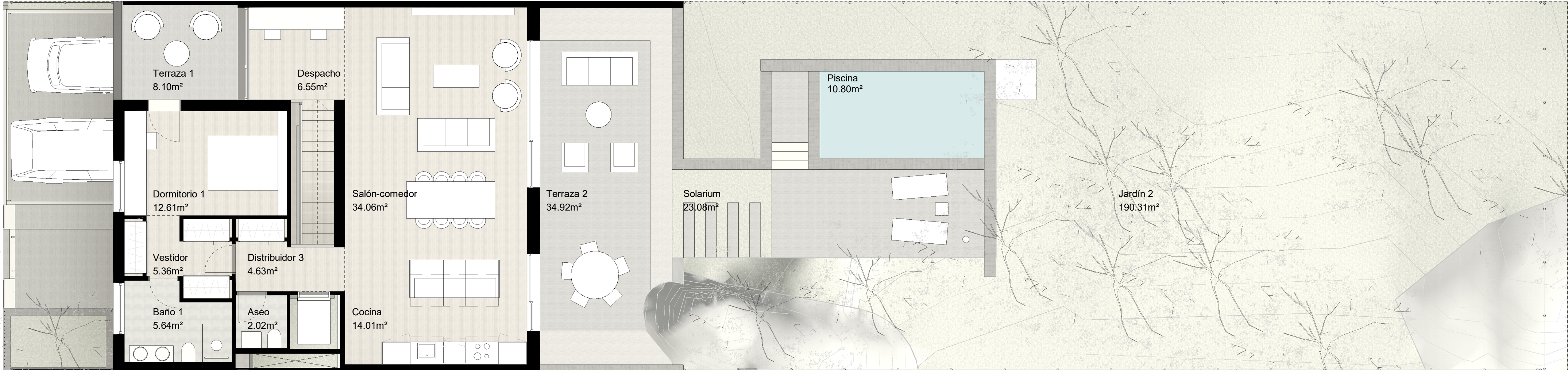
PLANTA PRIMERA
