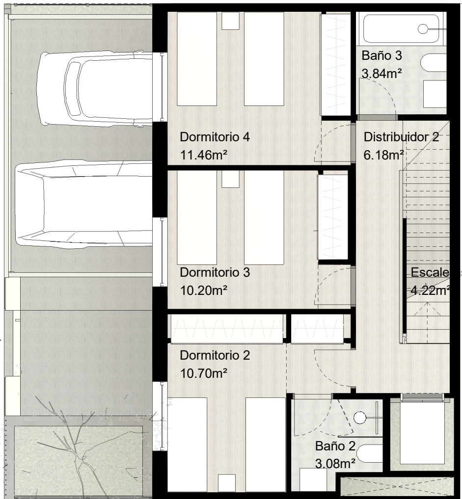
PLANTA BAJA
