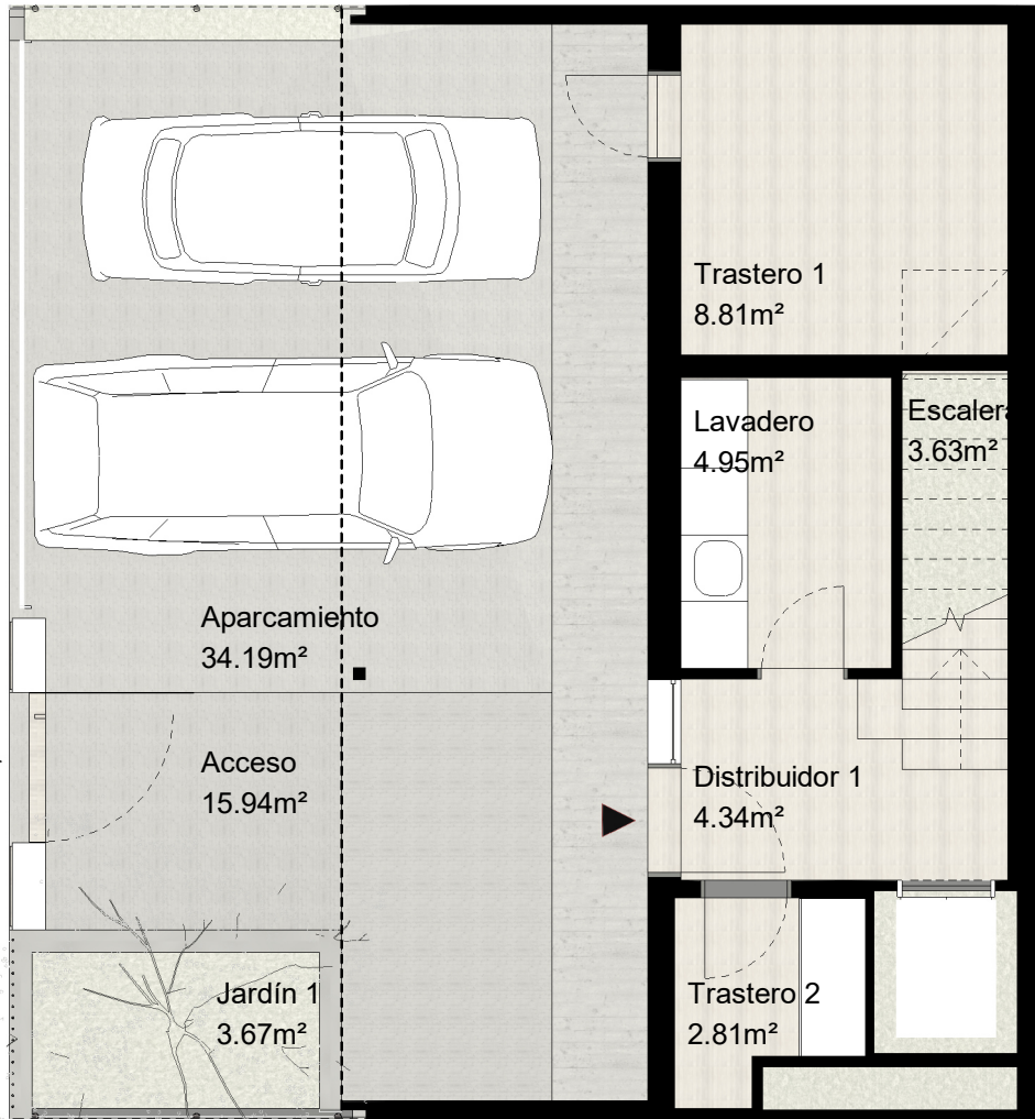
PLANTA SÓTANO
